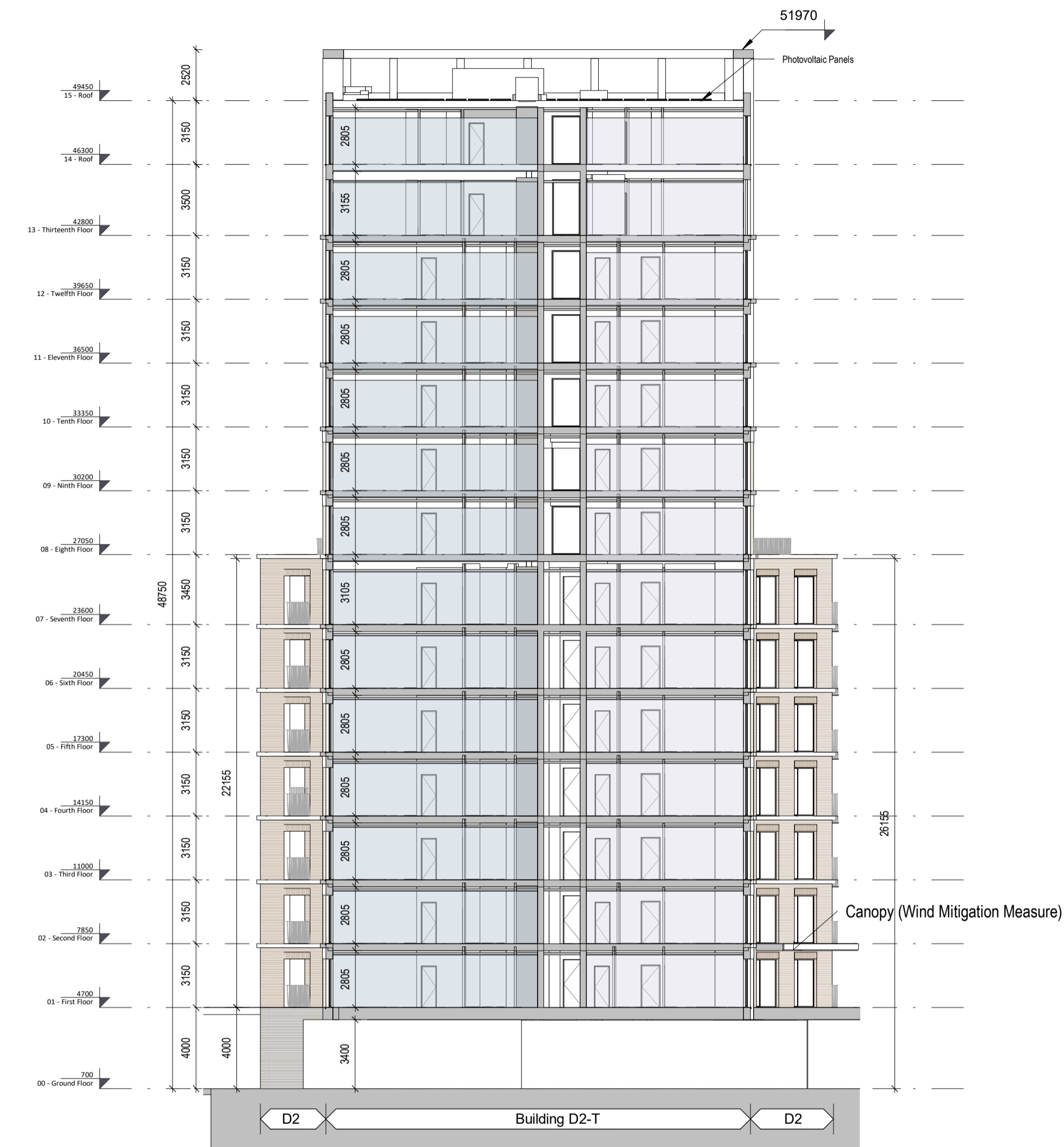
2 D2 & D2-T Section A-A 1:200
