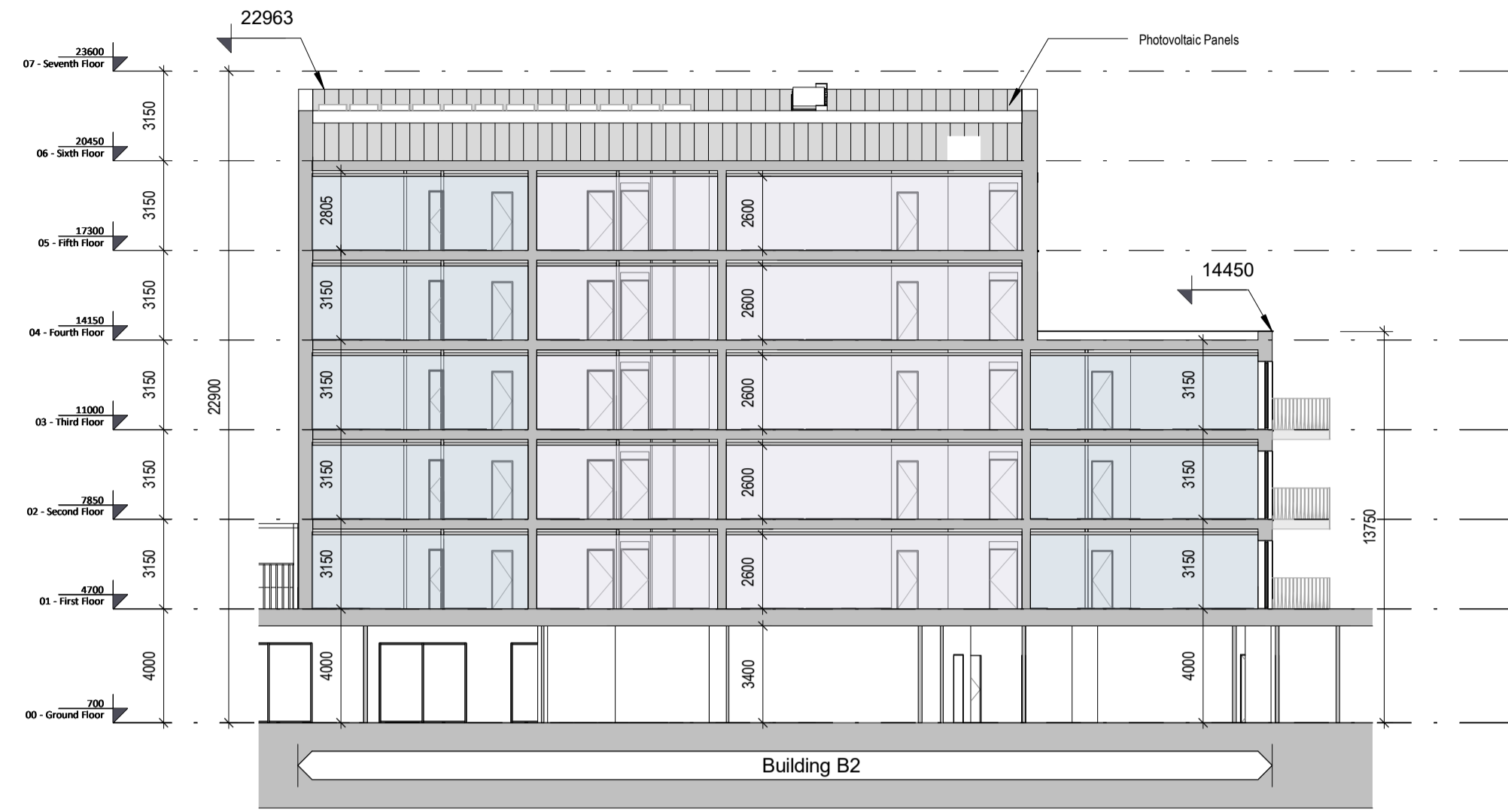
1 B2 Section A-A 1:200
